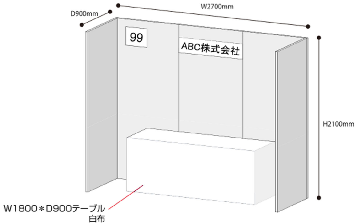
図2 展示ブース(1小間)イメージ図(案) ※ブースイメージは会場により変更されることがございます
