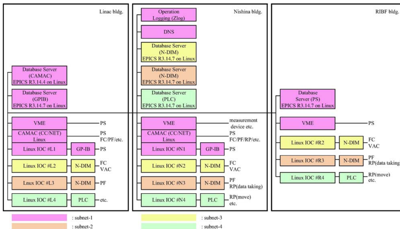
図1 RARF/RIBF制御系構成図
