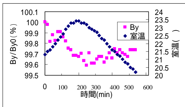
図 6 : 時間経過による磁場変化
