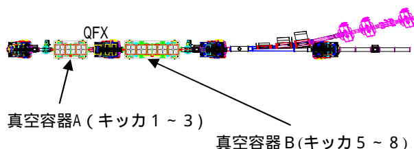
図1: 3 GeV RCS出射ビームライン
