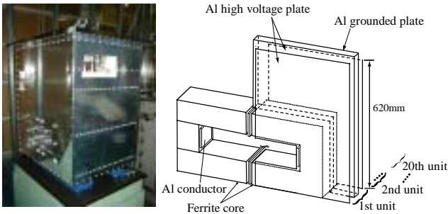
図2：キッカ電磁石全体、概念図
