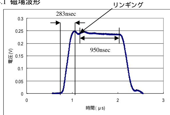
図4：測定磁場波形
