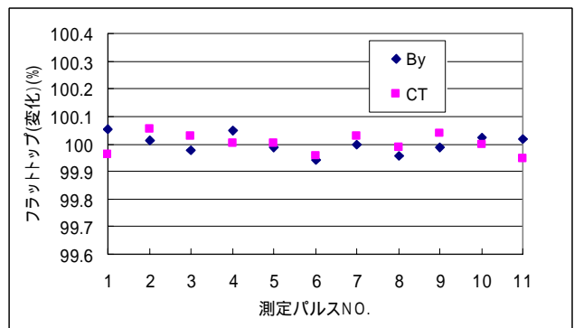
図5：パルス毎の安定度
