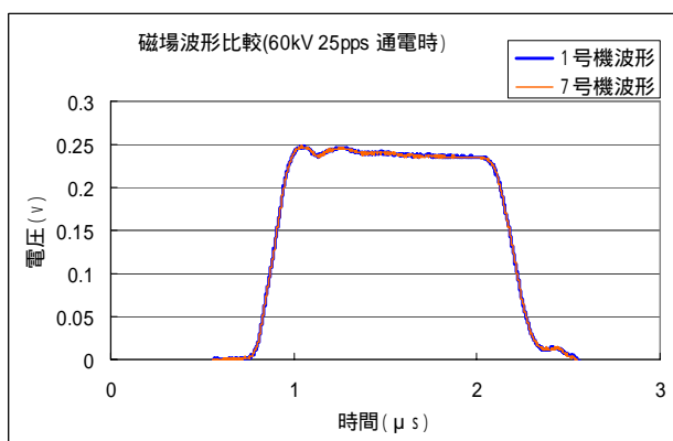
図 7 : 磁場波形比較
