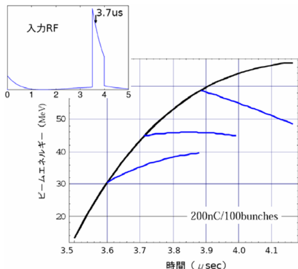
図3 加速管出口でのビームエネルギー
